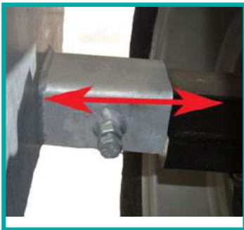
Asse regolabile in larghezza Axle adjustable in width
